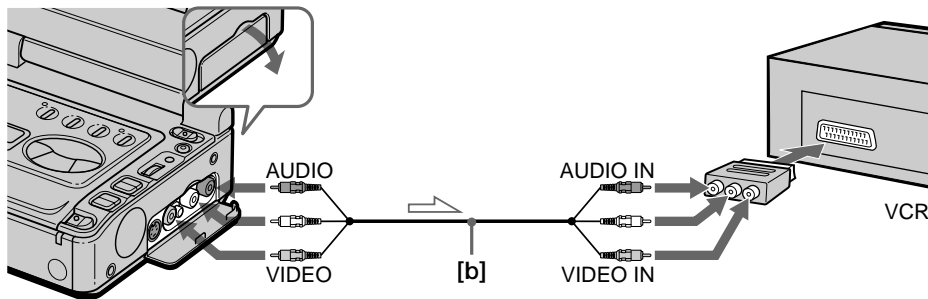
↔ : Signal flow / Передача сигнала
