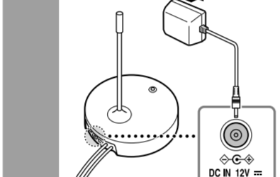
До розетки змінного струму
